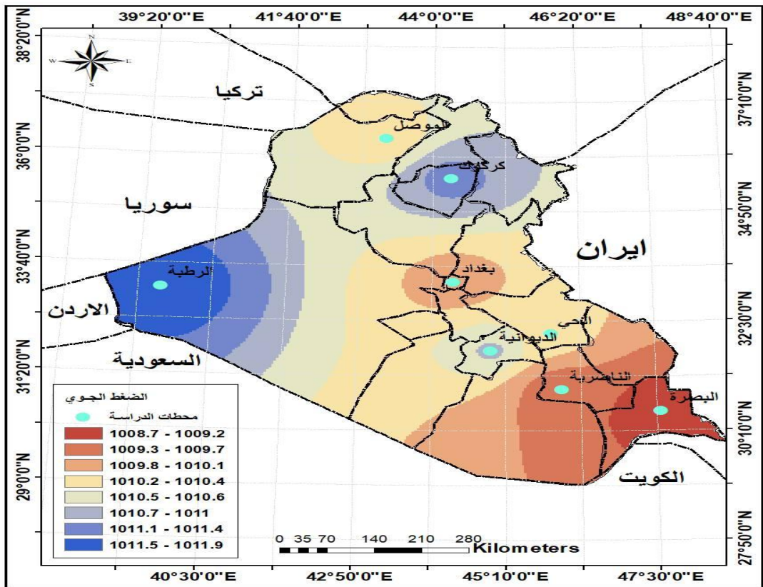
خريطة (2) معدل الضغط الجوي المصاحب للعواصف الرعدية للمدة (2023-2013)
