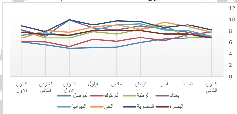
شكل (3) معدلات سرعة الرياح المصاحبة للعواصف الرعدية للمدة (2023-2013)
