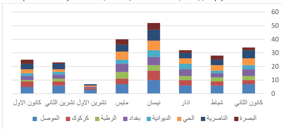
شكل (6) تكرارات البرد المصاحب للعواصف الرعدية للمدة (2023-2013)
