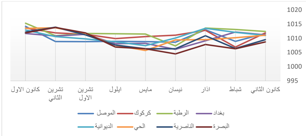
شكل (2) معدل الضغط الجوي المصاحب للعواصف الرعدية للمدة (2023-2013)
