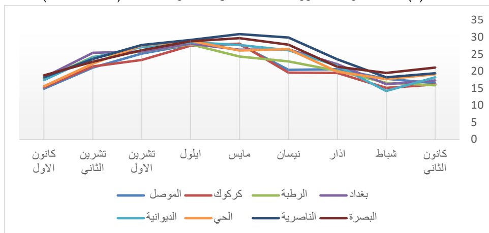
شكل (4) معدلات درجات الحرارة المصاحبة للعواصف الرعدية للمدة (2023-2013)
