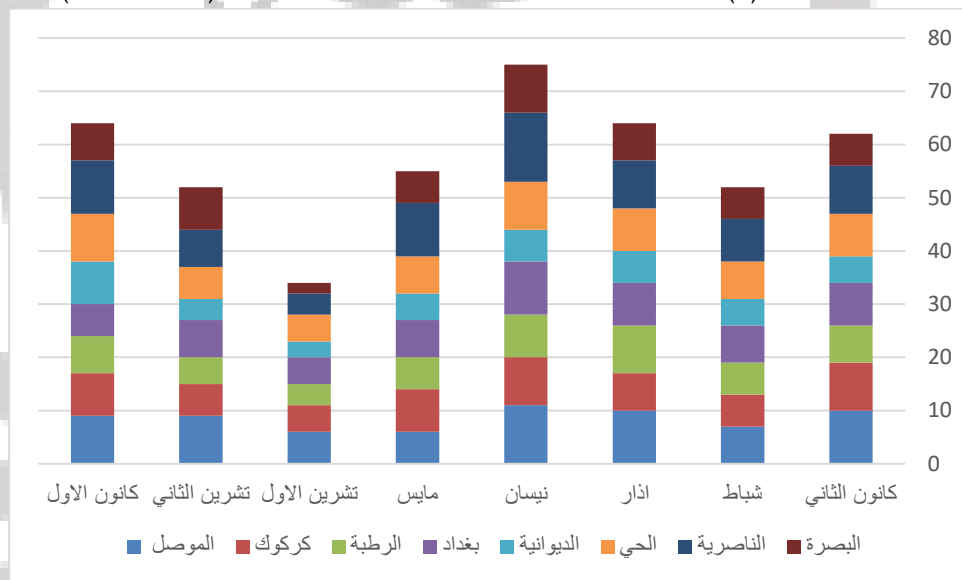
شكل (5) تكرارات الأمطار المصاحبة للعواصف الرعدية للمدة (2023-2013)
