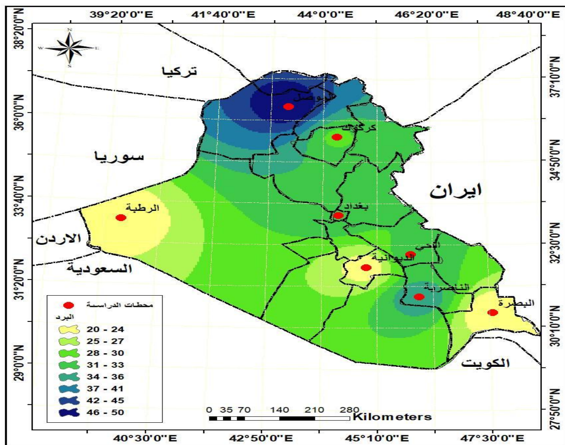
خريطة (6) تكرارات البرد المصاحب للعواصف الرعدية للمدة (2023-2013)
